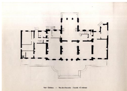
Plan du rez-de-chaussée du petit château en 1913, après agrandissement A.M.N.S.S., Cote 2 Z 354
